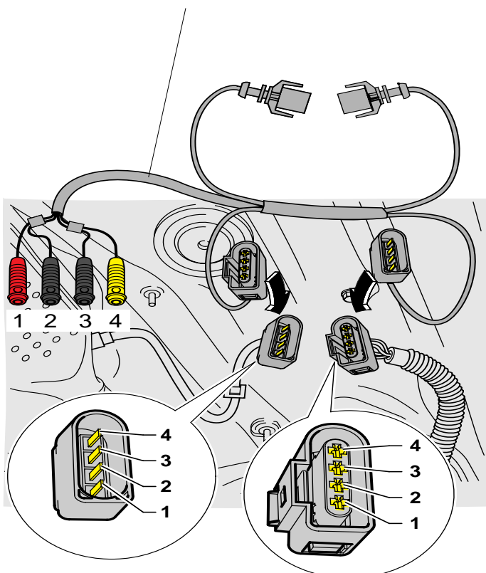
Lambda-Sondenadapter VAS 5103
