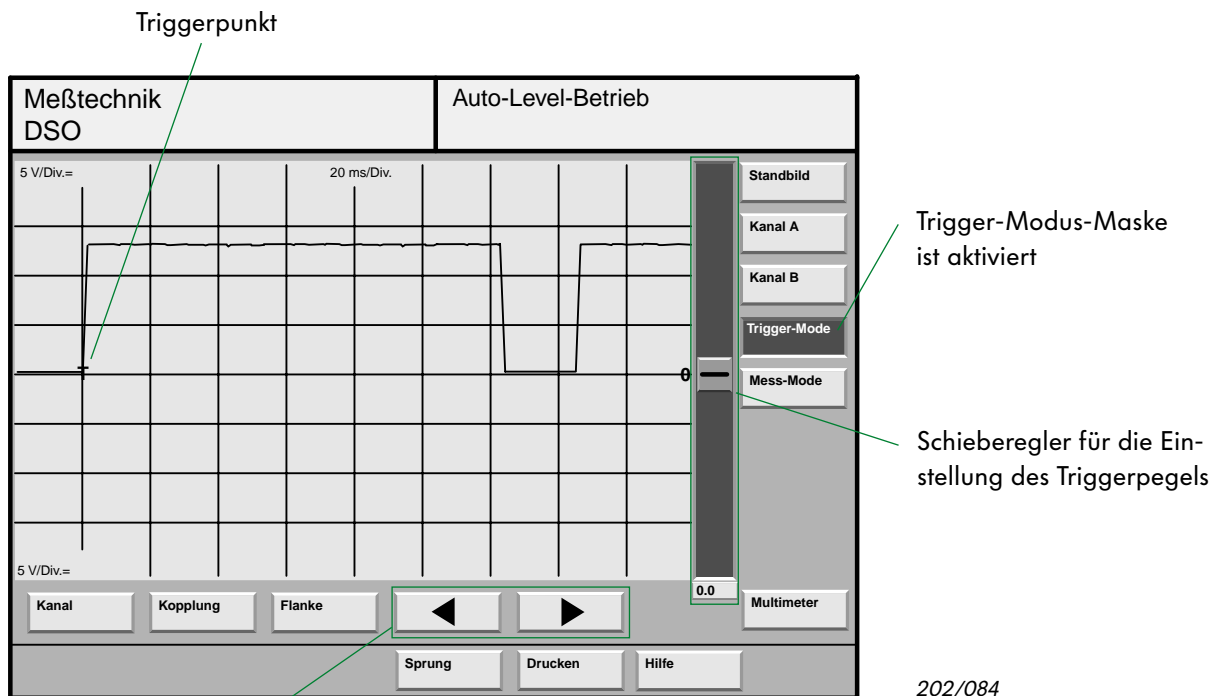
„Pfeil“-Schaltflächen zum Verschieben des Triggerpunktes
