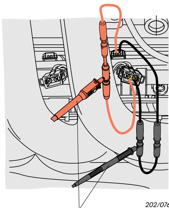
DSO-Meßkabel
